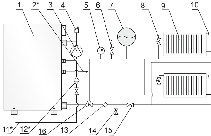
Мал. 10. Приклад двотрубної закритої системи опалення з примусовою циркуляцією.
